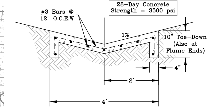
Typical Storm Flume N.T.S.
