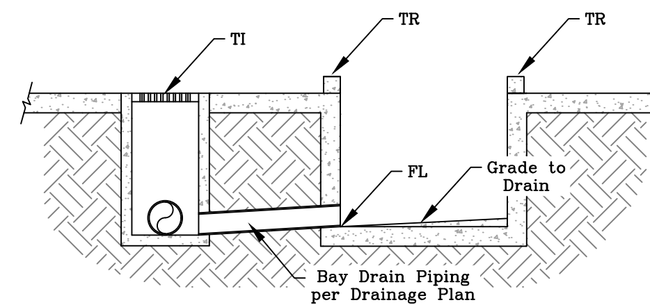
Bay Drain - Section A-A N.T.S.
