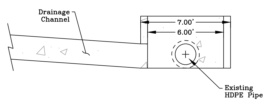
Weir Tie-In Assembly Section A-A N.T.S.
