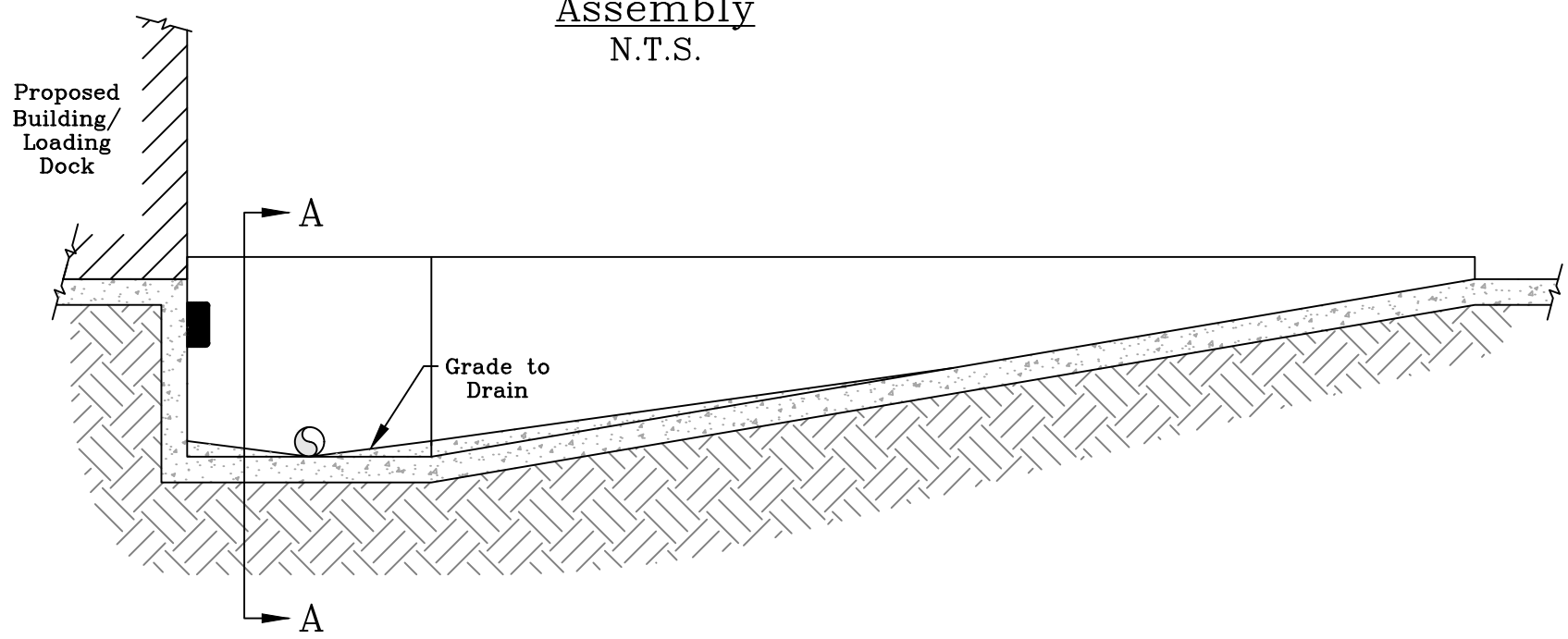
Bay Drain - Profile N.T.S.
