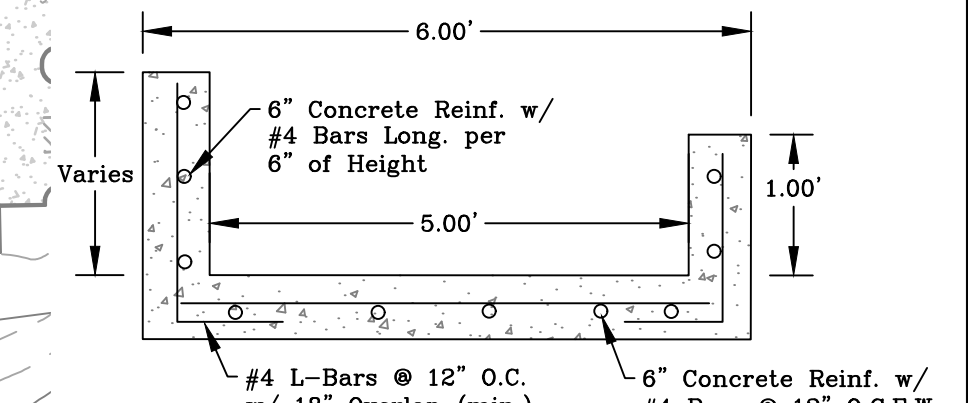
Drainage Channel N.T.S.
